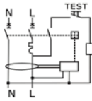
1 Polo + Neutro (a sinistra) 1 Modulo
