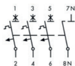
3 Poli + Neutro 4 Moduli
